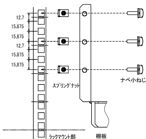
＜正面側＞ 固定位置詳細
