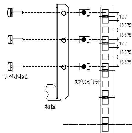
＜背面側＞ 固定位置詳細
