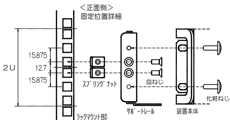
固定位置詳細図
